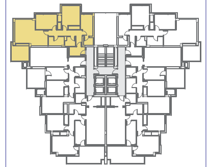
EDIFICIO I PLANTA TIPO
